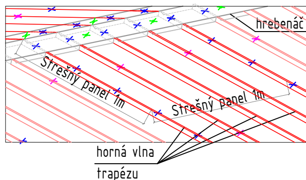
D4 - Detail kotviacich prvkov na 1m x 1m
