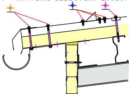
D1 - Kotvenie dažďového zvodového systému
