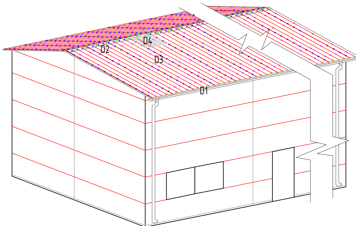
D1 - Kotvenie dažďového zvodového systému
