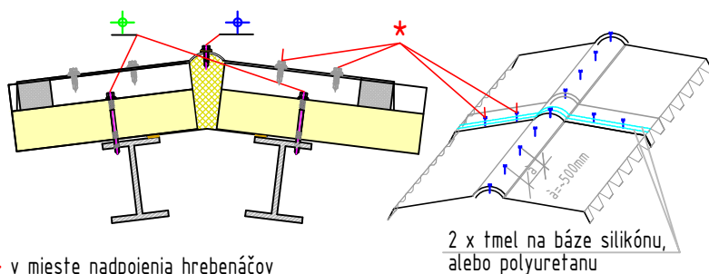
D2 - Detail kotviacich prvkov v hrebeni
